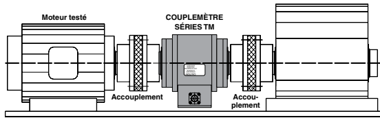
Couplèmetre suspendu
