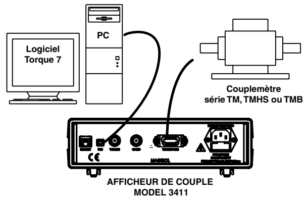
Configuration du système avec un PC Couplèmetre avec afficheur modèle 3411 et logiciel Torque 7
