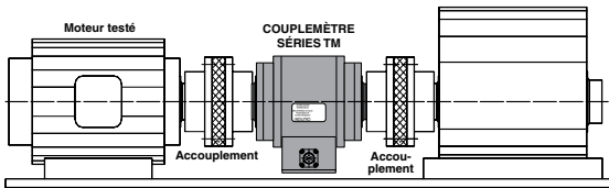
Couplemètre suspendu (pour des essais à petite vitesse, utiliser des accouplements simples pour raccourcir l'unité d'entraînement)
