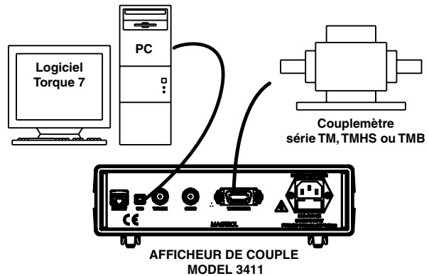
Configuration du système avec un PC Couplemètre avec afficheur modèle 3411 et logiciel Torque 7
